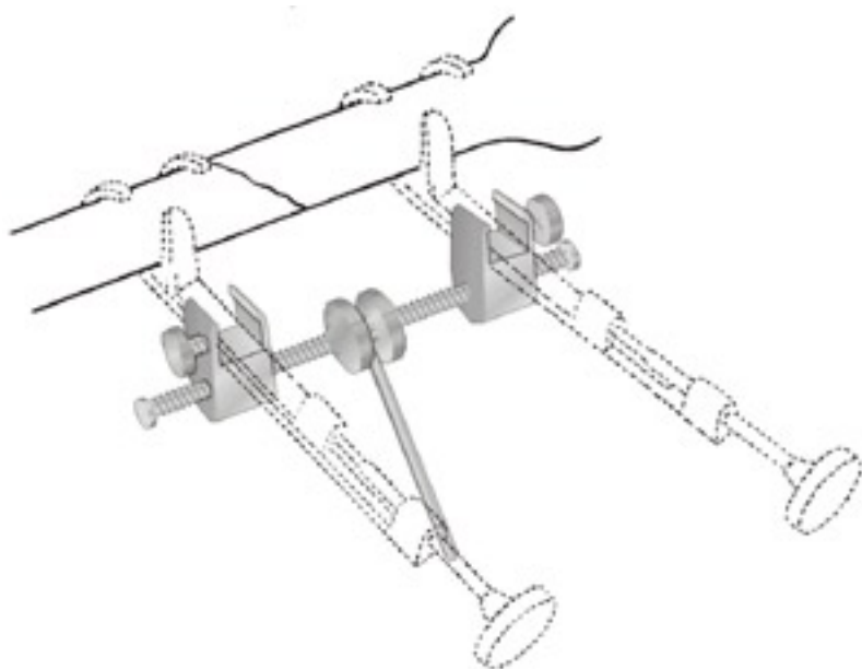
Gerster Distraktionsklammer KF.420.15 passend für Lowman Knochenhalteklammern
